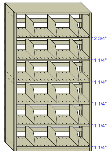
R1 42"W x 12"D H=76 1/4"
