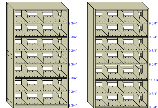
R1 42"W x 12"D H=76 1/4"
